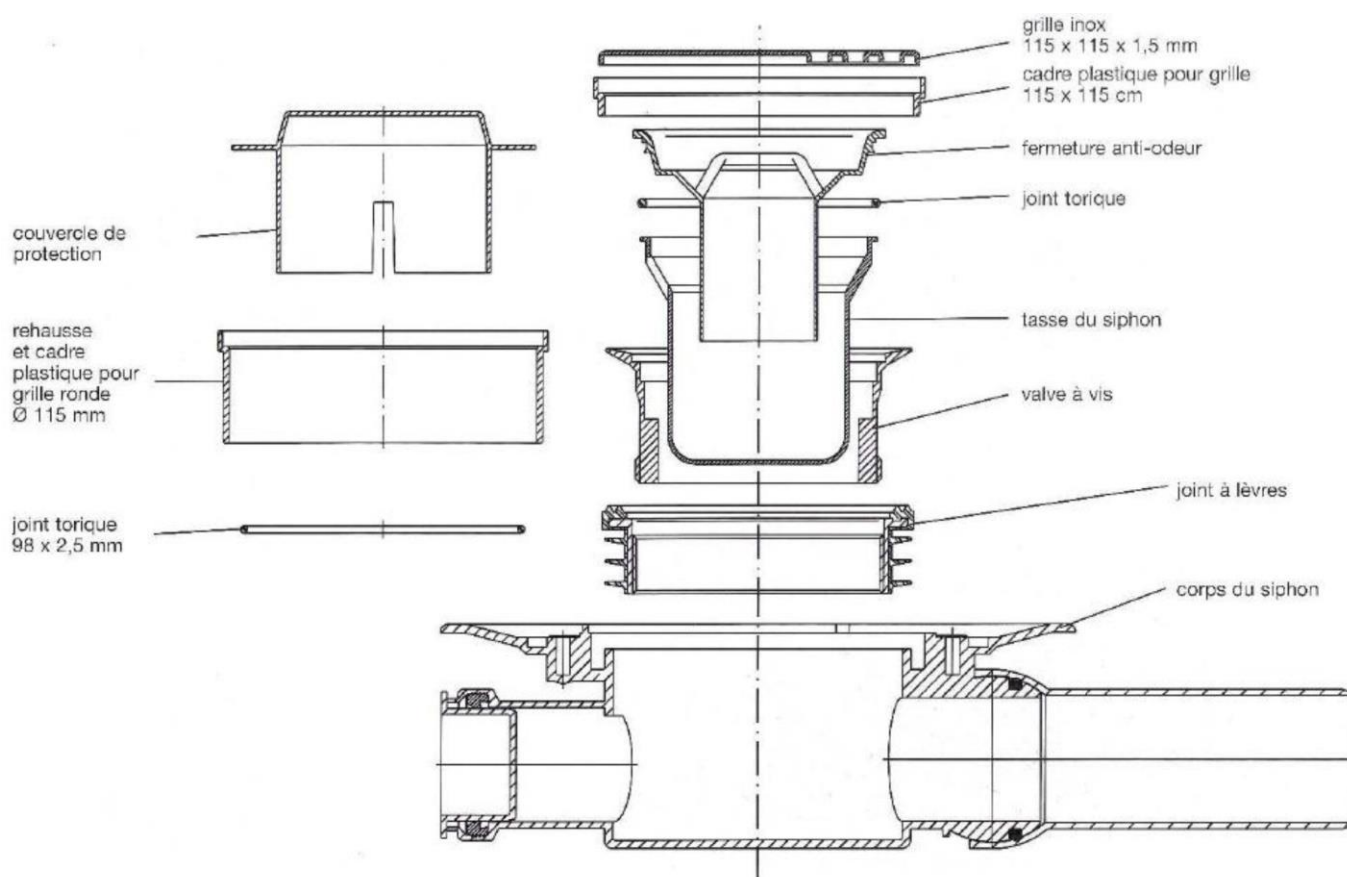
Fig 7 : vue en coupe d'un siphon Fundo Primo ou Fundo Ligno plus
