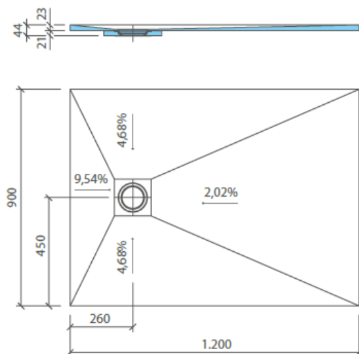
Figure 5 : plan Fundo Ligno en 1200x900
