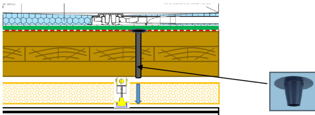
Fig 9 : vue en coupe du principe de réalisation d'un détecteur de fuite sous plancher massif CLT
