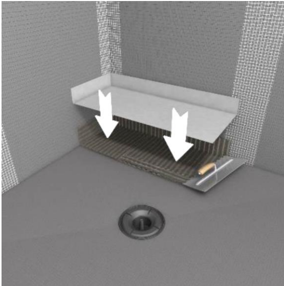
Figure 17 : collage au SEL wedi 520 de la natte d'étanchéité Fundo Plano sur la partie comblée
