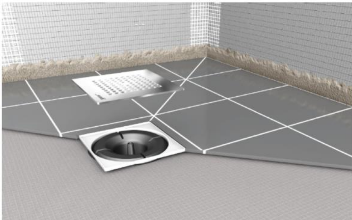
Figure 22 : mise en œuvre du revêtement céramique ( receveur Fundo Plano )
