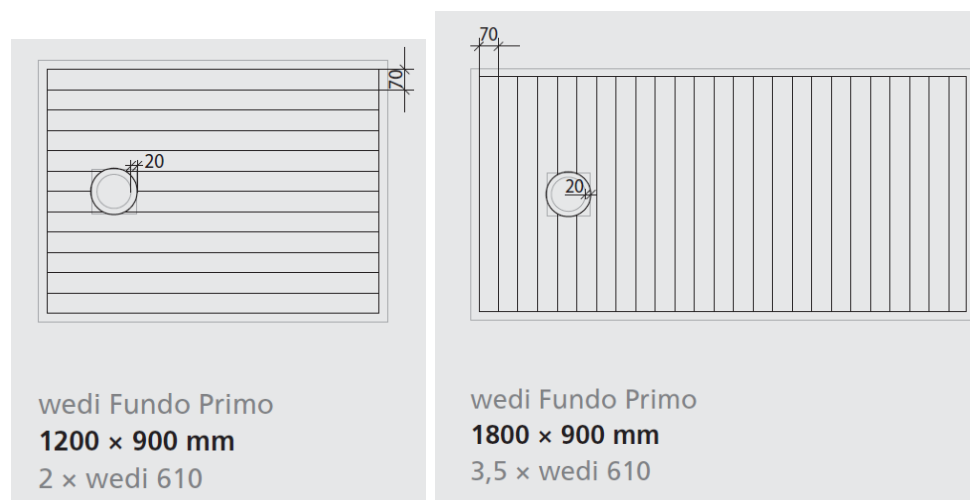
Figure 23 : exemples de répartition de la colle wedi 610 pour receveur Fundo
