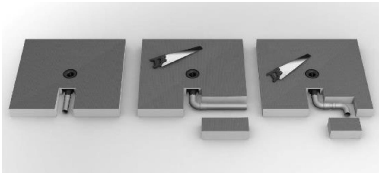
Figure 15 : exemples de découpes du receveur Fundo plano en fonction de la position de la canalisation d'évacuation d'eau
