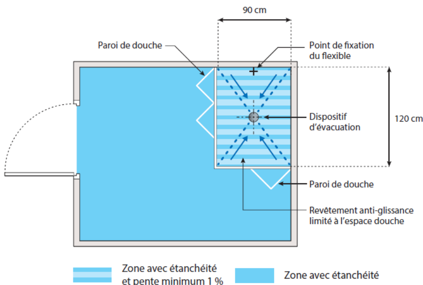
Figure 1 : douches zéro ressaut cloisonnées
