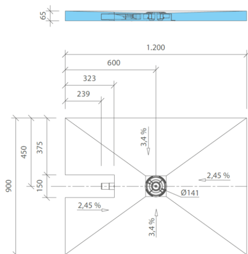
Figure 6 : plan Fundo Plano en 1200x900
