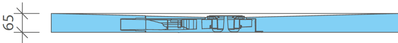
Figure 8 : vue en coupe d'un siphon Fundo Plano intégré dans le receveur
