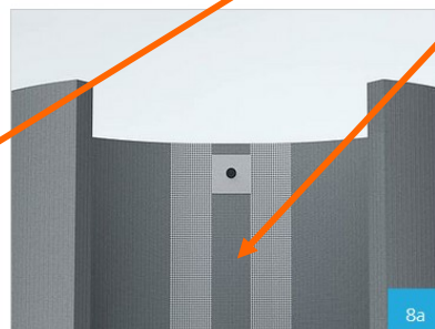
Pour la version Fundo Trollo libero avec armature encastrée, étancher les perforations avec de la colle polymère wedi 610 et avec des collerettes d'étanchéité wedi Tools appropriées.
